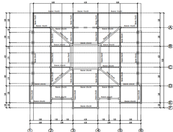
Gambar 5. Denah Balok Dan Kolom Masjid Baiturrahim Serampon
