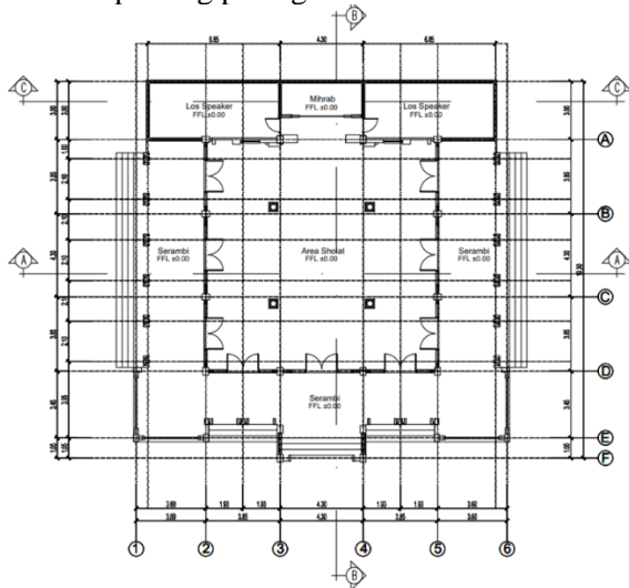
Gambar 3. Denah lantai satu masjid baiturrahim serampon
