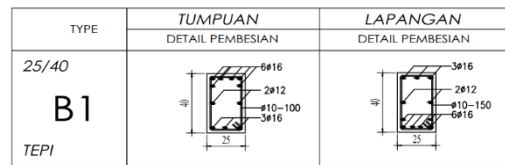
Gambar 4. Detail Penulangan Struktur Portal Beton Bertulang Masjid Baiturrahim Serampon
