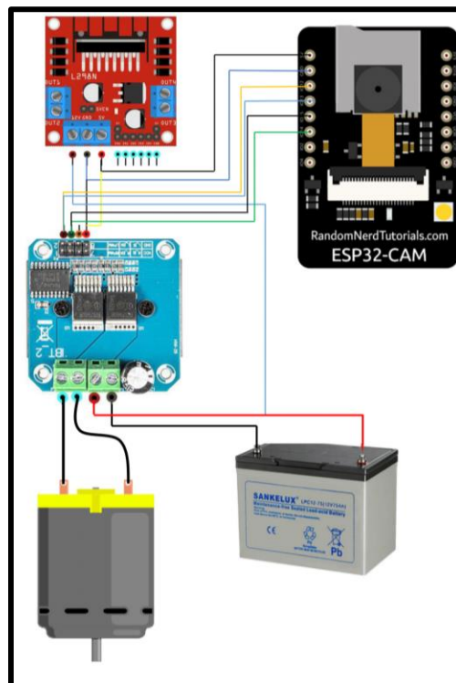
Gambar 2.3 Rangkaian Komponen.
