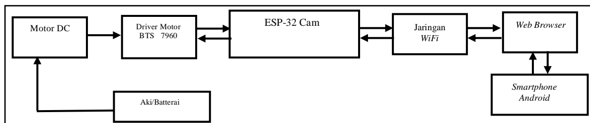
Gambar 2.2 Diagram Blok.
