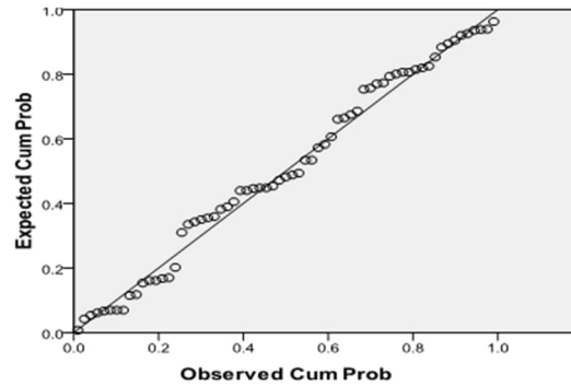
Gambar 1. Hasil Uji Normalitas Menggunakan Grafik P-Plot
