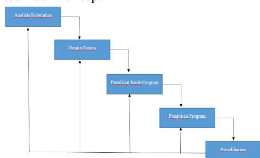
Gambar 2 Tahapan Metode.
