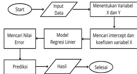
Gambar 2. Alur Implementasi Metode Regresi Linier
