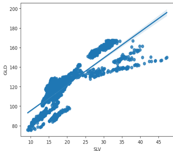
Gambar 3. Grafik Regresi Linier pada Data Training
