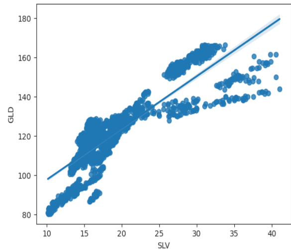
Gambar 4. Grafik Regresi Linier pada Data Training Single Variable
